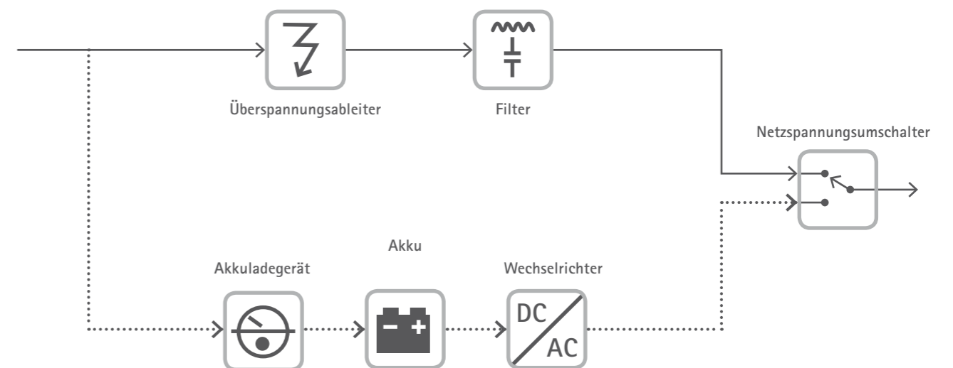
Abb. 5.1: Standby- oder Offline-USV (Klasse 3)
