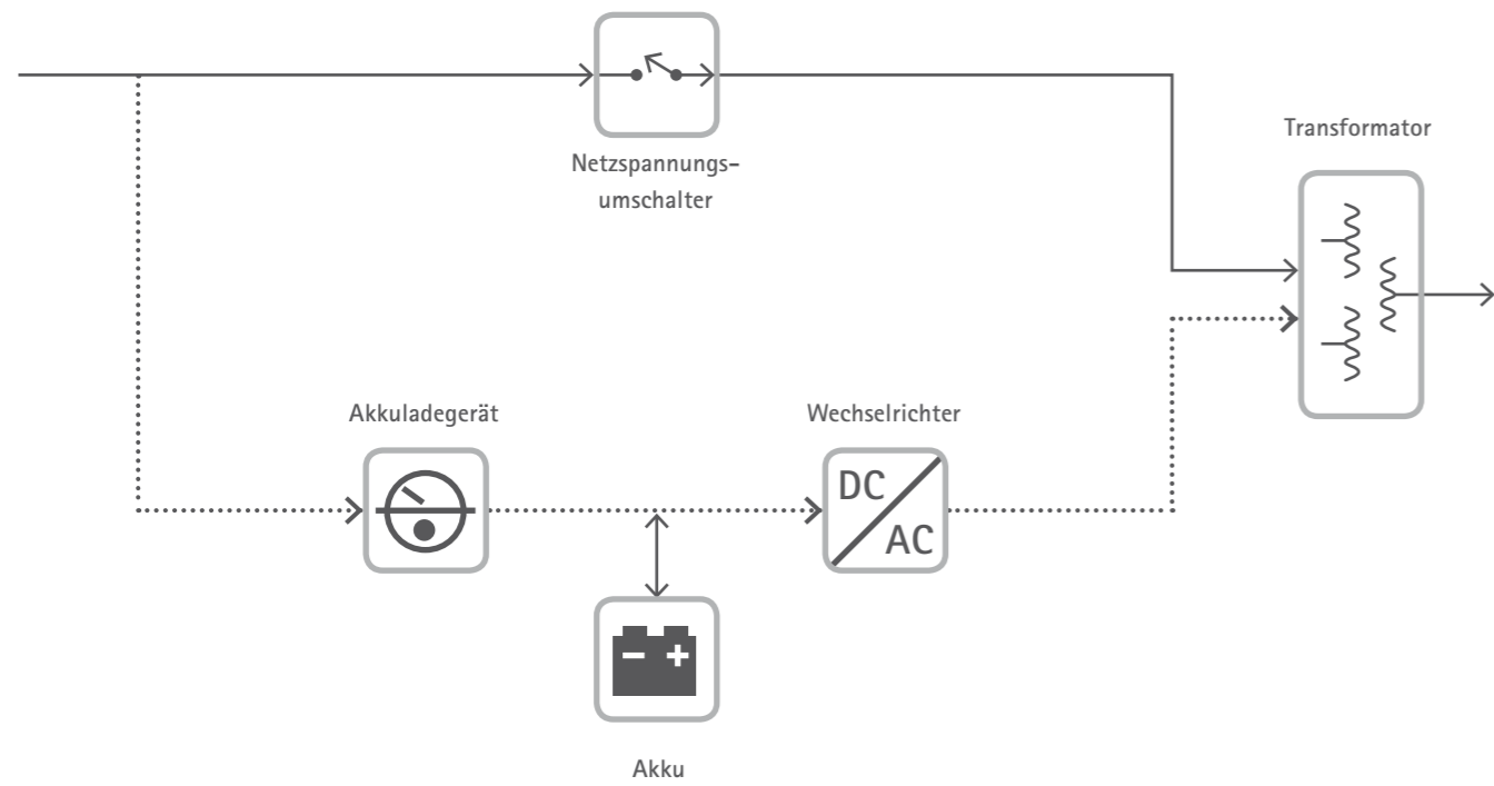
Abb. 5.2: Netzinteraktive-USV (Klasse 2)
