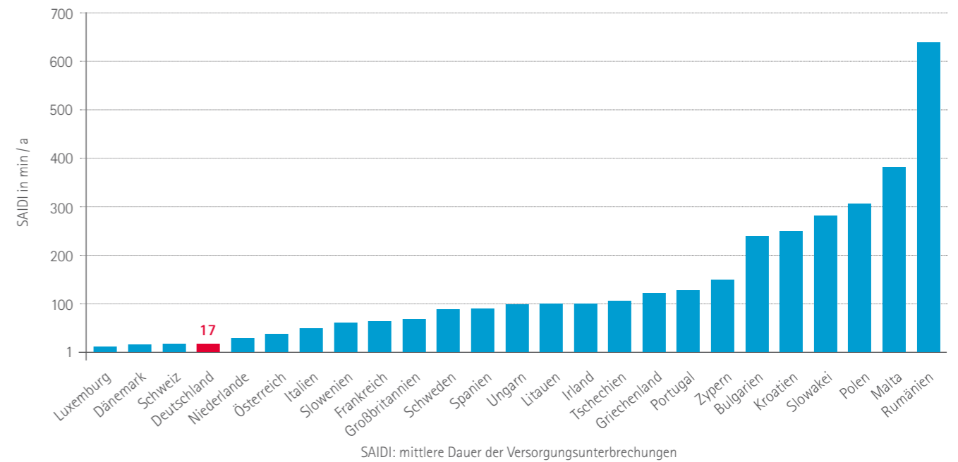
Abb. 2.5: Mittlere SAIDI-Werte 2006-2014 im europäischen Vergleich, eigene Darstellung nach [25] und [40]
