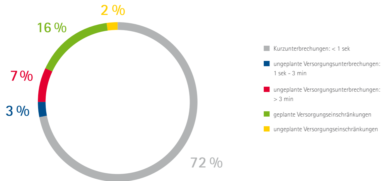
Abb. 2.4: Aufteilung der Versorgungsstörungen nach Vorfalldtyp, eigene Darstellung nach [23]
