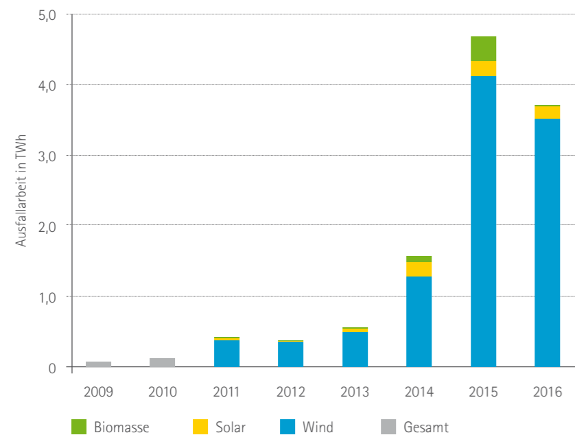
Abb. 1.1: Ausfallarbeit durch Einspeisemanagement in Deutschland 2009 bis 2016 nach den Monitoringberichten der Bundesnetzagentur [10]
