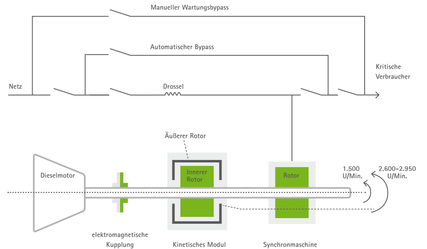
Abb. 5.5: Prinzipielle Darstellung eines dieseldynamischen USV-Systems
