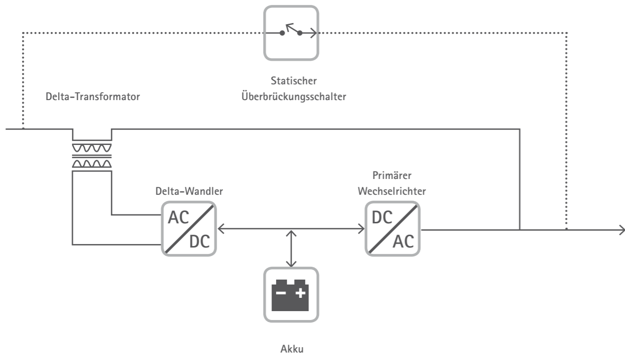
Abb. 5.3: Online-USV (Klasse 1)
