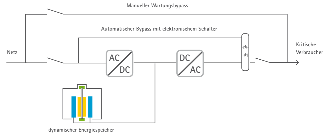
Abb. 5.4: Prinzipieller Aufbau einer dynamischen USV-Anlage
