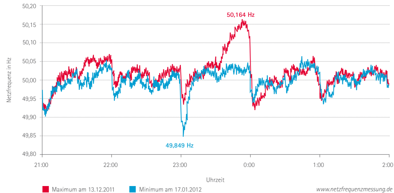
Abb. 2.2: Netzfrequenz mit Maximum und Minimum [19]
