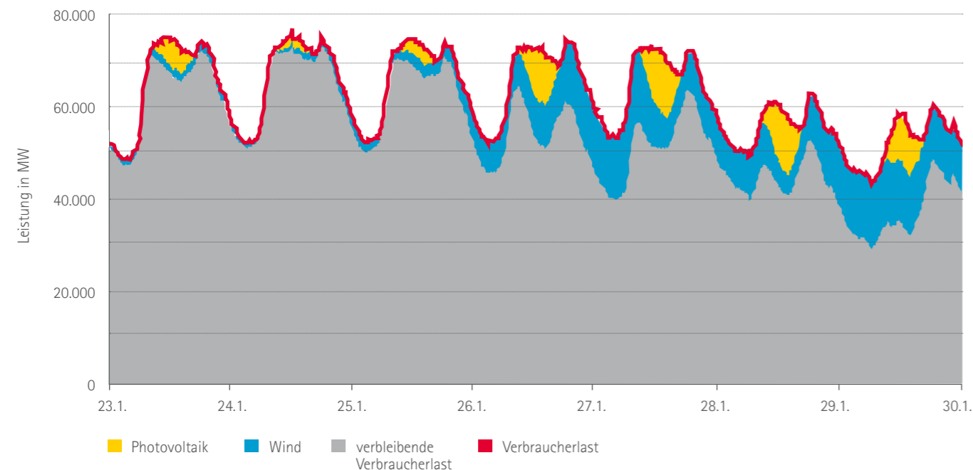
Abb. 2.1: Einspeisecharakteristik Photovoltaik und Windenergie in der Woche vom 23.01. bis 30.01.2017, eigene Darstellung nach [15] und [16]
